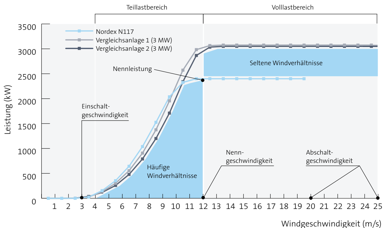
Leistungskennlinien verschiedener Windenergieanlagen im Vergleich
